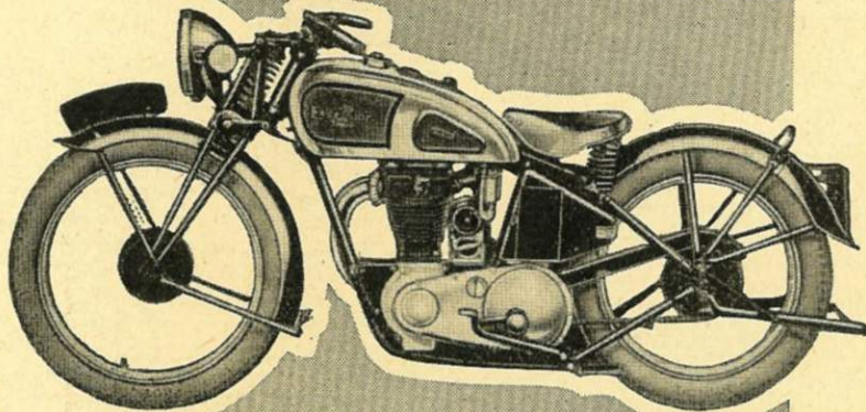
250 c.c. O.H.V. "NORSEMAN"
