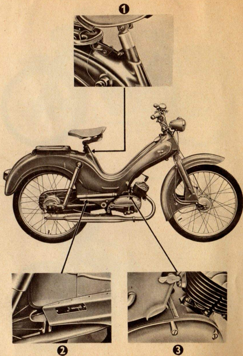
Motor- 3 und Fahrgestell-Nummer 1 sowie Typenschild 2 der DKW Hummel
