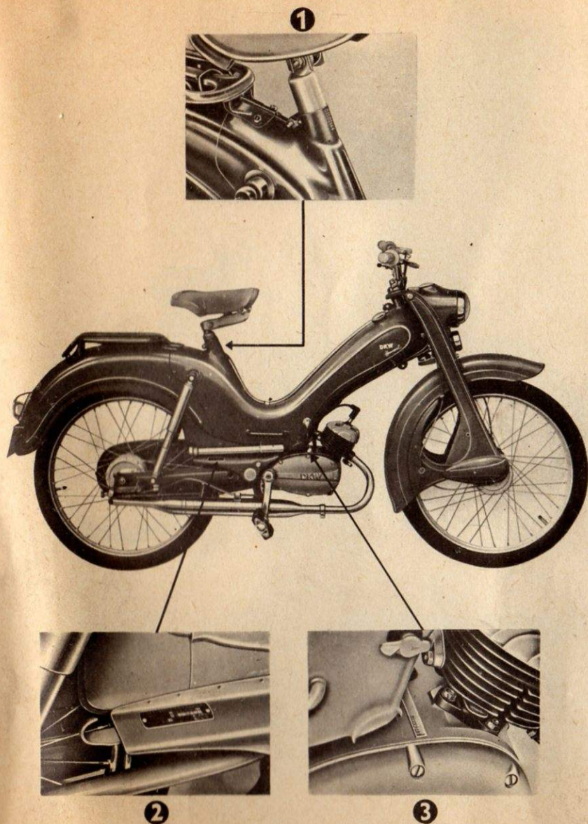
Motor- ③ und Fahrgestell-Nummer ① sowie Typenschild ② der DKW Hummel
